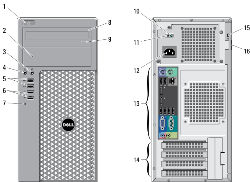
Figura 1. Vista anteriore e posteriore
