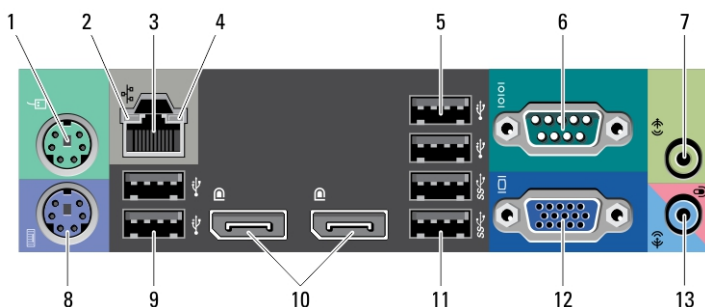
Figura 2. Vista del pannello posteriore
